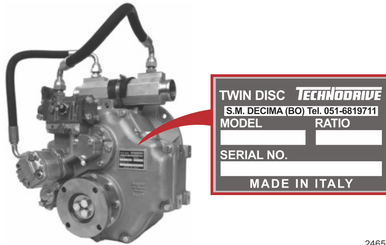
Plaque signalétique de la transmission Technodrive TM 485-A
